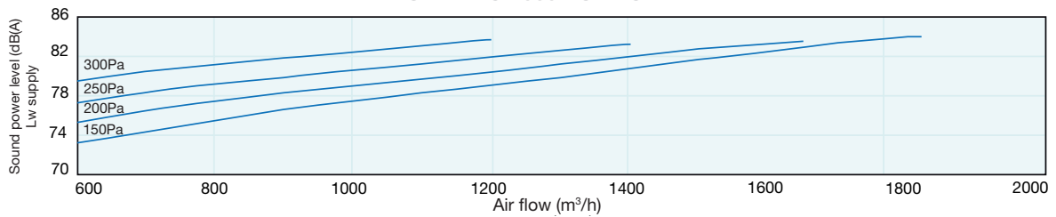
VORT NRG 2000 EC - EC EH
