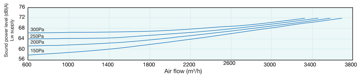
VORT NRG 3000 ECR - ECR EH
