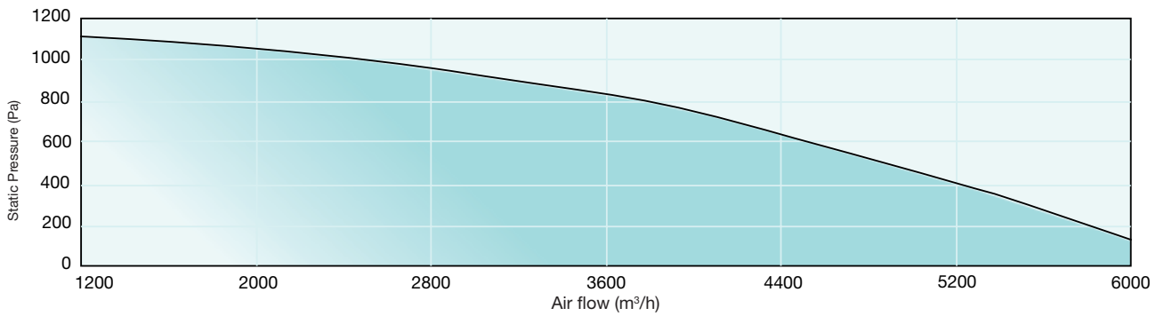
VORT NRG 6000 EC - EC EH
