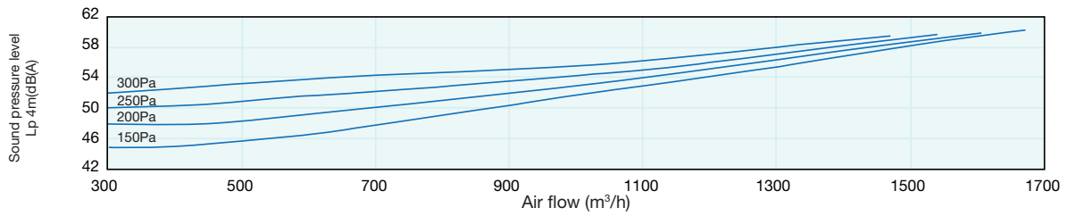
VORT NRG 2000 ECR - ECR EH
