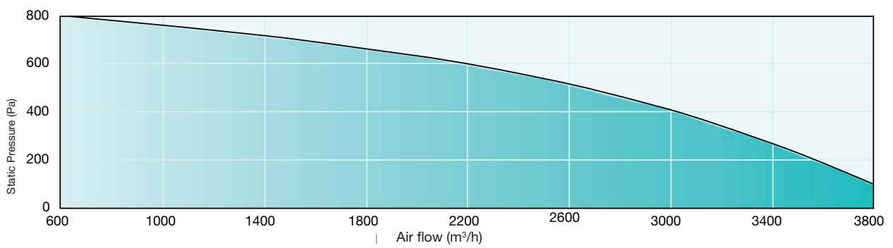
VORT NRG 3000 ECR - ECR EH
