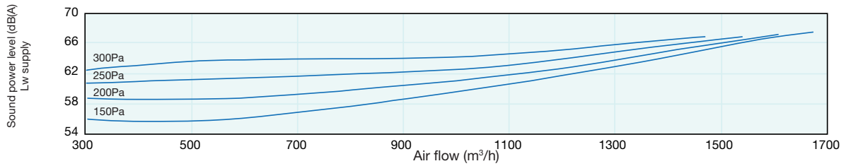
VORT NRG 800 ECR - ECR EH
