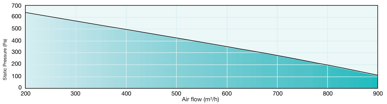
VORT NRG 800 ECR - ECR EH
