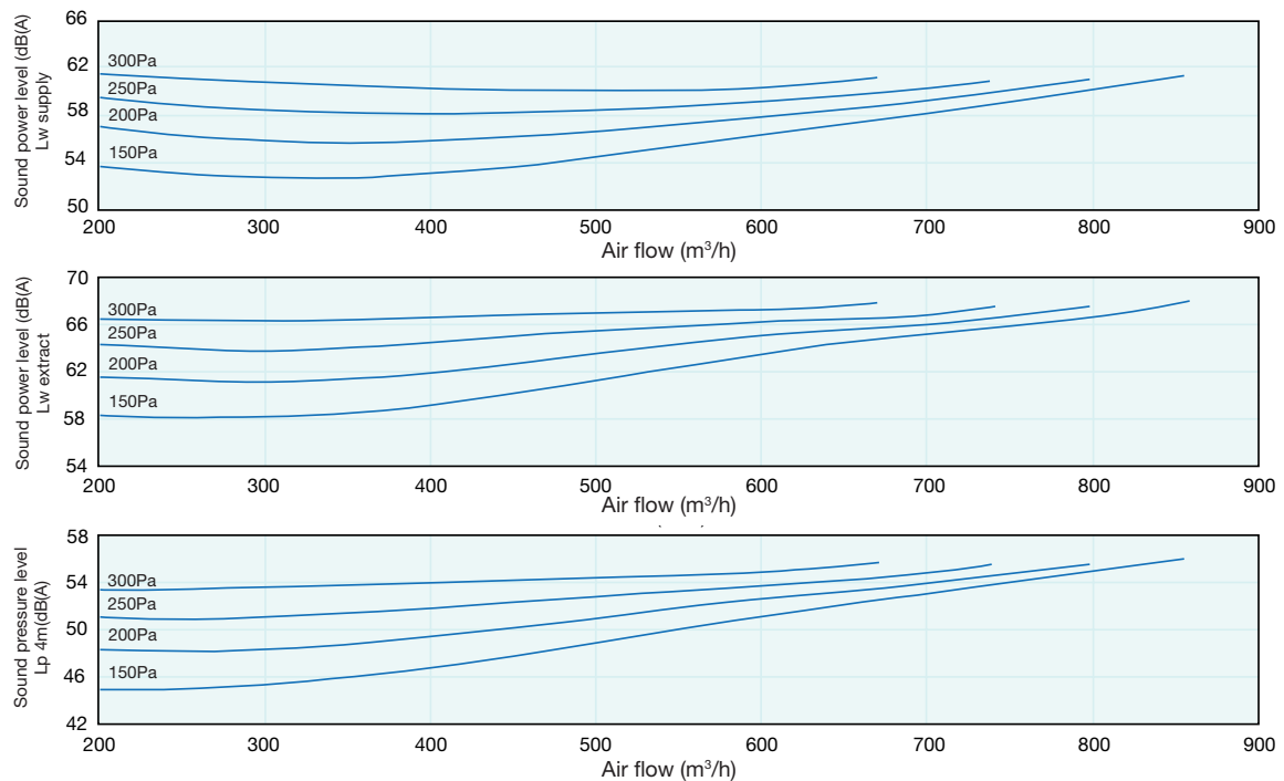
VORT NRG 1500 ECR - ECR EH
