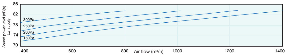
VORT NRG 1500 EC - EC EH
