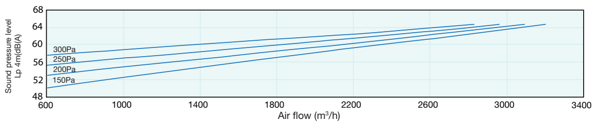
VORT NRG 3000 ECR - ECR EH
