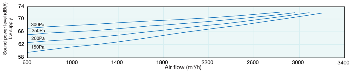
VORT NRG 2500 ECR - ECR EH
