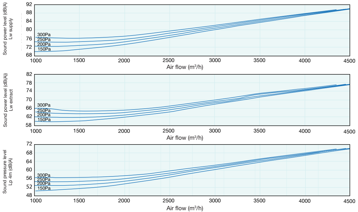
VORT NRG 6000 EC - EC EH
