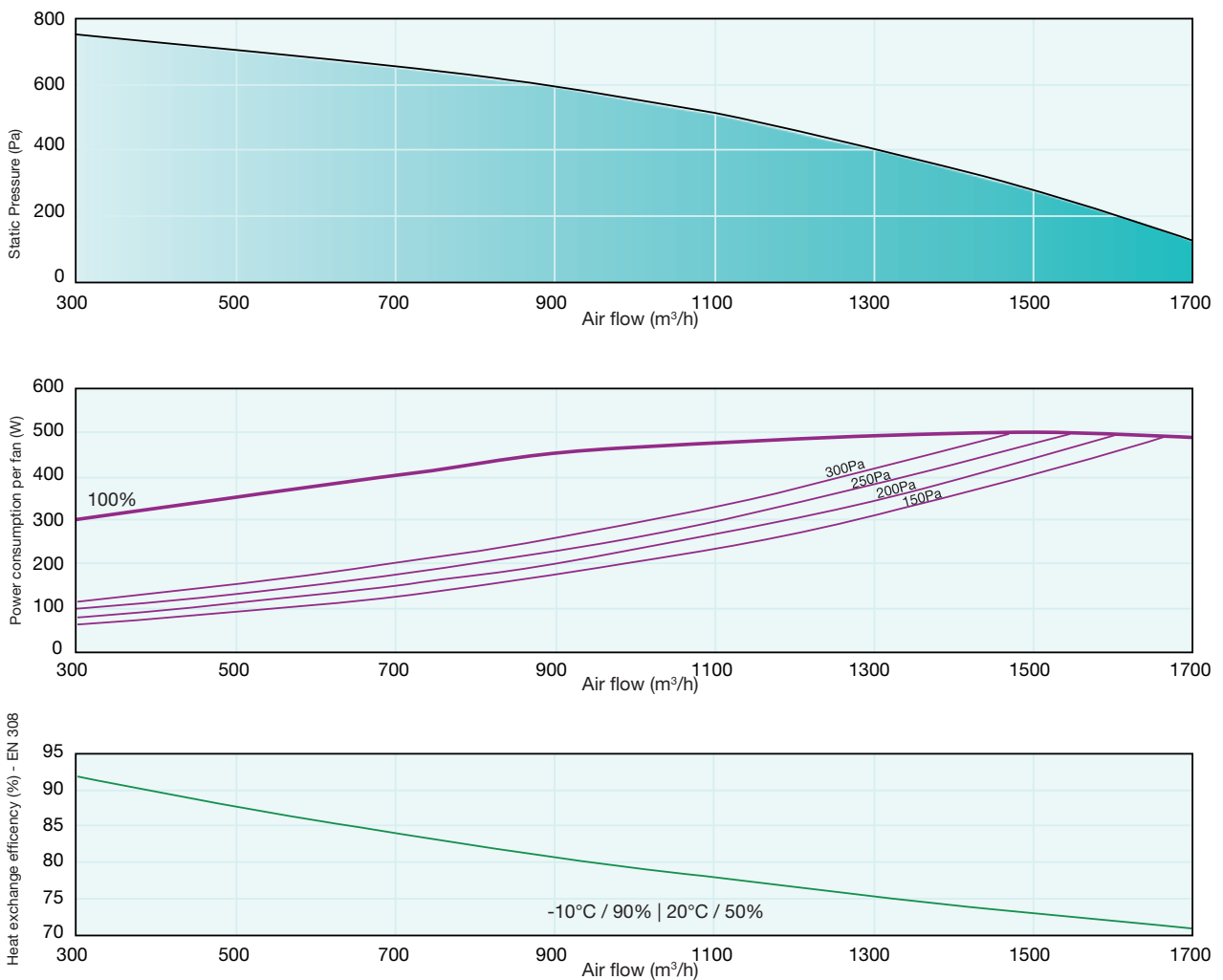
VORT NRG 1500 ECR - ECR EH
